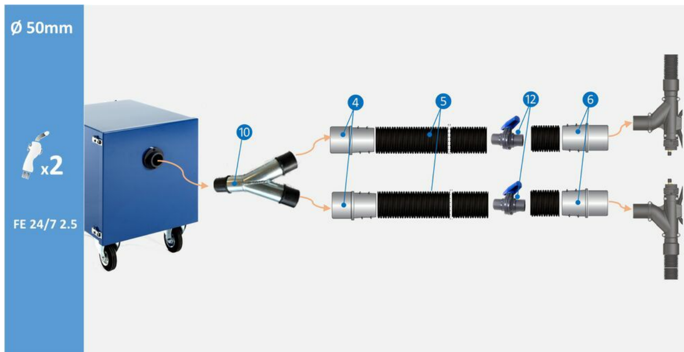
Tilbehørskonfigurasjon for to brukere, 50mm sveiseapparattilkobling. (10) Forgrening 50/50/50, art.nr. 55999420 (4) Slangekobling M50-50P, art.nr. 55999416 (5) Slange PE-51 L=5m, art.nr. 55999412 (12) Kuleventil 51 mm, art.nr. 55999421 (6) Slangekobling F50-50P, art.nr. 55999417
