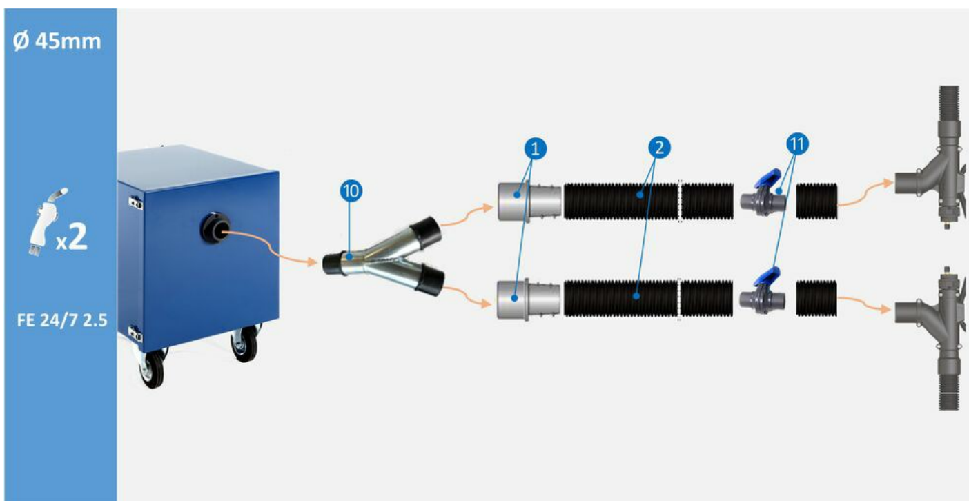
Tilbehørskonfigurasjon for to brukere, 45 mm sveiseapparattilkobling. (10) Forgrening 50/50/50, art.nr. 55999420 (1) Slangekobling M50-44P, art.nr. 55999418 (2) Slange Superflex Ø 45 mm svart 5 m, art.nr. 55999411 (11) Kuleventil 44 mm, art.nr. 55999422
