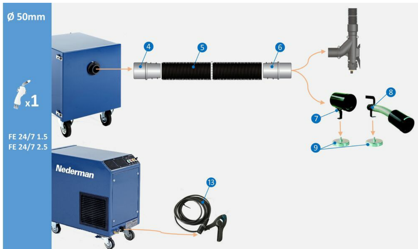
Tilbehørskonfigurasjon for én bruker, 50mm sveiseapparattilkobling. (4) Slangekobling M50-50P, art.nr. 55999416 (5) Slange PE-51 L=5 m, art.nr. 55999412 (6) Slangekobling F50-50P, art.nr. 55999417 (7) Munnstykke CWN-S 105/50 lyddemper, art.nr. 55999415 (8) Munnstykke CWN-S 105/50L lyddemper, art.nr. 55999414 (9) Magnetisk fot for munnstykke CWN-S, art.nr. 55999419 (13) Sensorklemme med plugg for automatisk start/stopp, art.nr. 55999410
